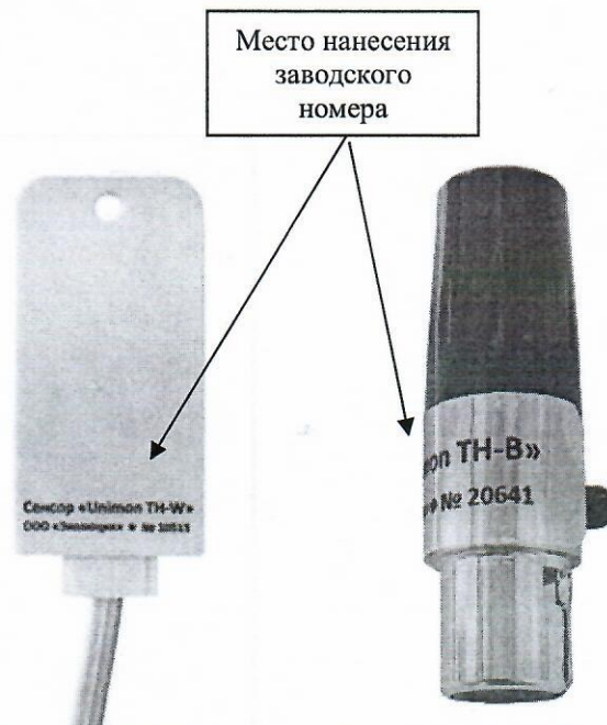
Рисунок 2 – Общий вид датчиков исполнения «Unimon TH-B»
